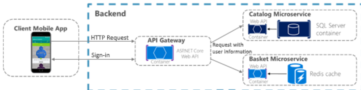
图 11-1. 使用 API 网关中心化验证
