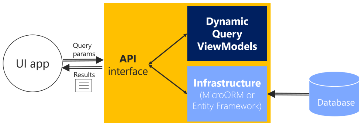
图9-3. 一个CQRS 微服务中最简单的查询
