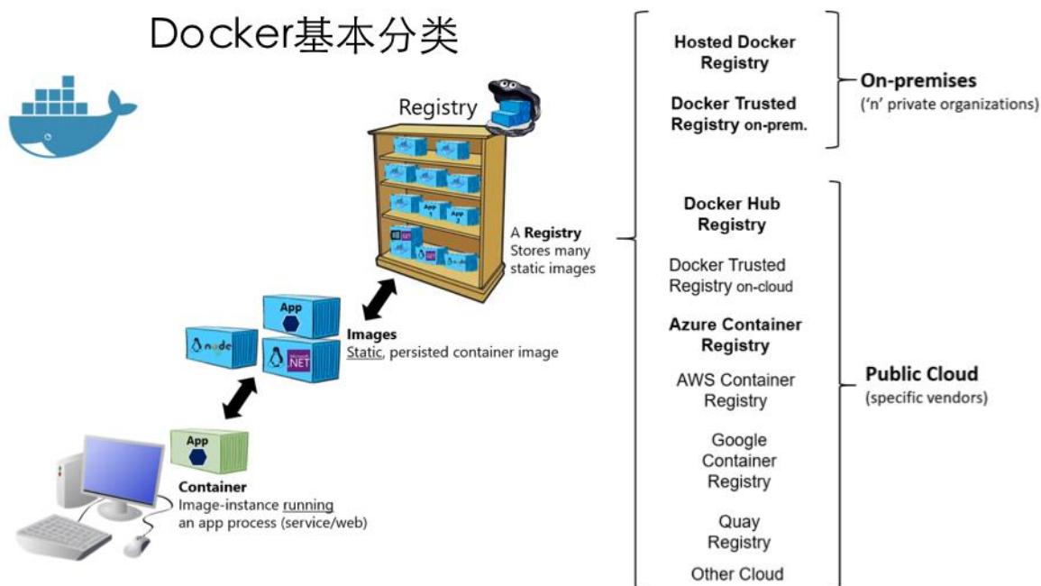
图 2-4. Docker 术语和概念的分类
