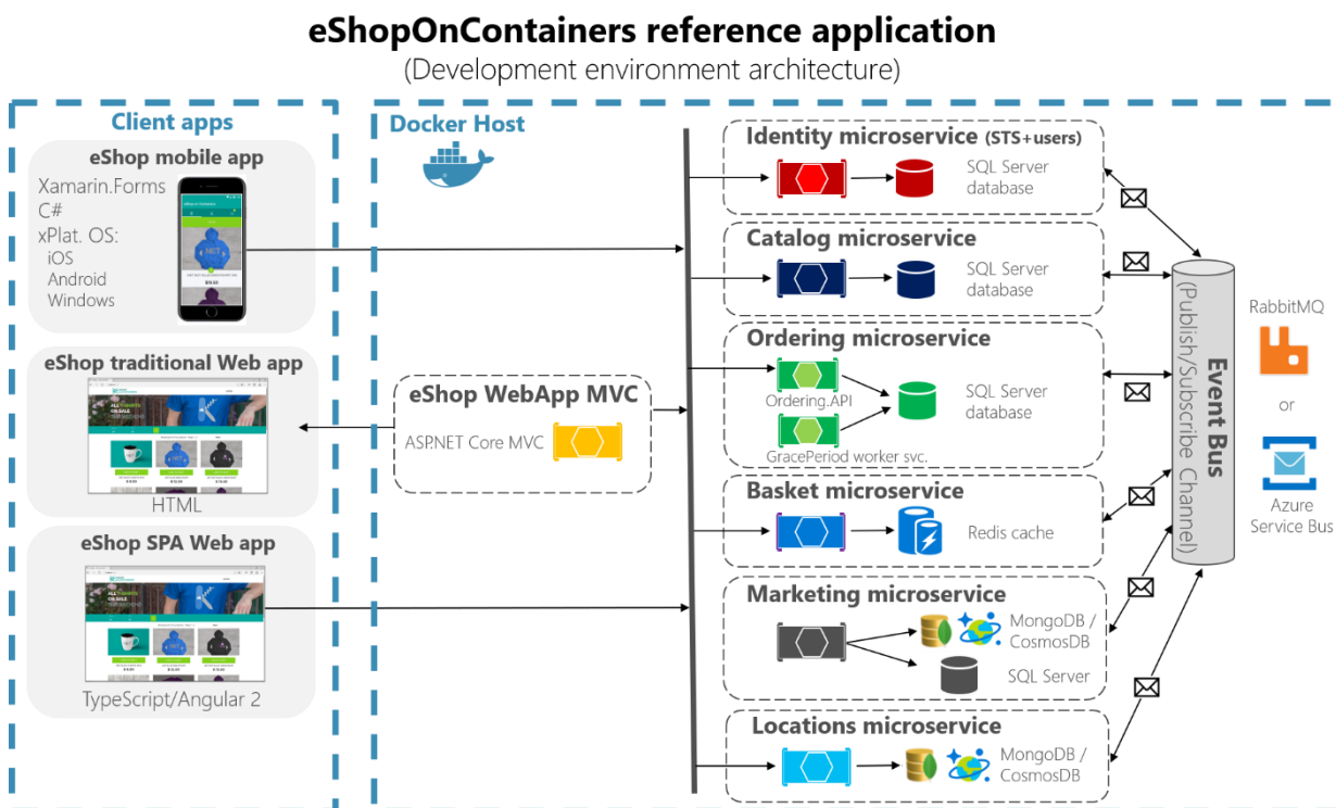
图 8-1. 针对开发环境的 eShopOnContainers 示例应用程序架构
