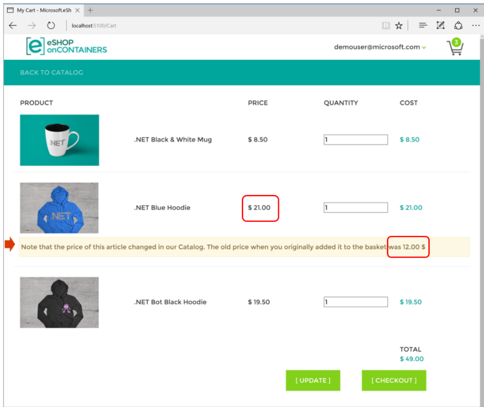
图 8-24. 通过集成事件通信来显示购物篮中的项目价格变动
