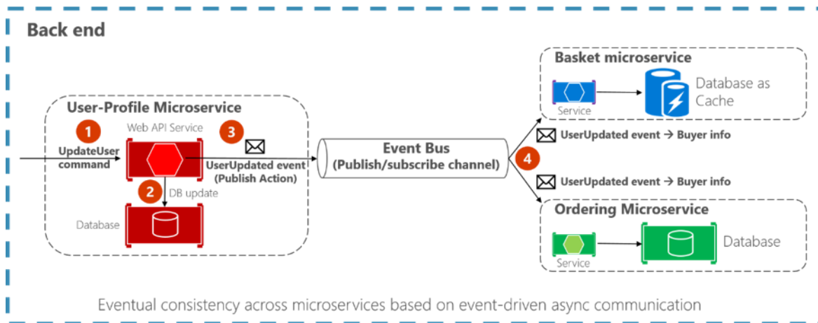
图 4-19. 异步事件驱动消息通信
