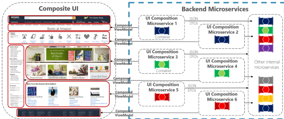
图 4-21. 由后端微服务生成的组合式界面应用示例
