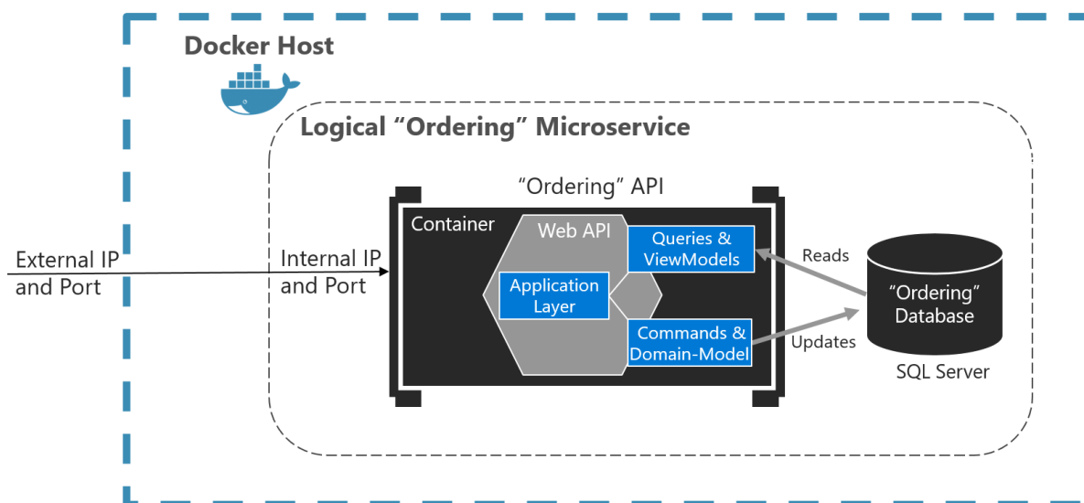
图9-2. 基于简化的CQRS和DDD的微服务
