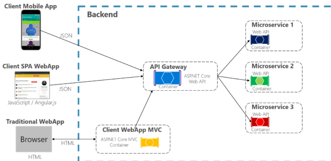
图 4-13. 在微服务架构中使用 API 网关模式
