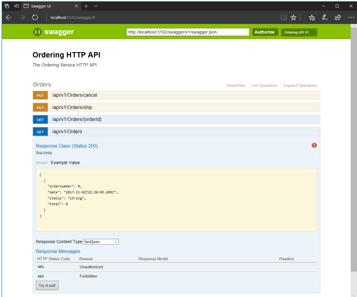
图9-5. Swagger UI 展示一个 Web API 的响应类型和可能的 HTTP 状态码
