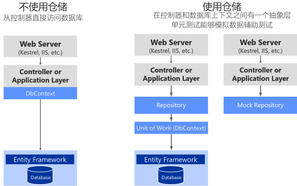
图9-18. 使用自定义仓储与使用纯 DbContext
