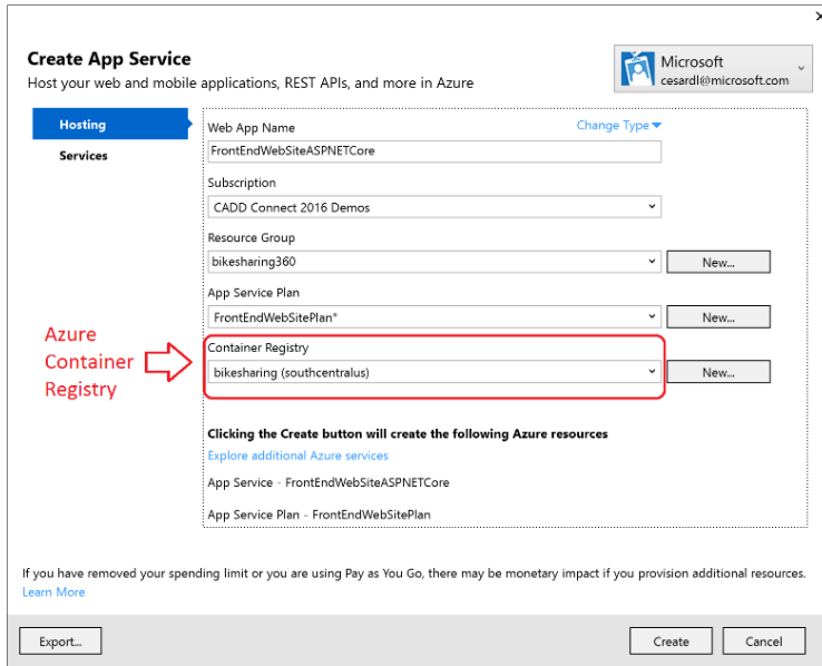
图 4-4. 从 Visual Studio 发布一个单容器应用到 Azure 应用服务
