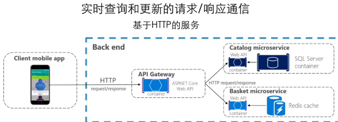
图4-16. 使用 HTTP 请求/响应通信（同步或异步）
