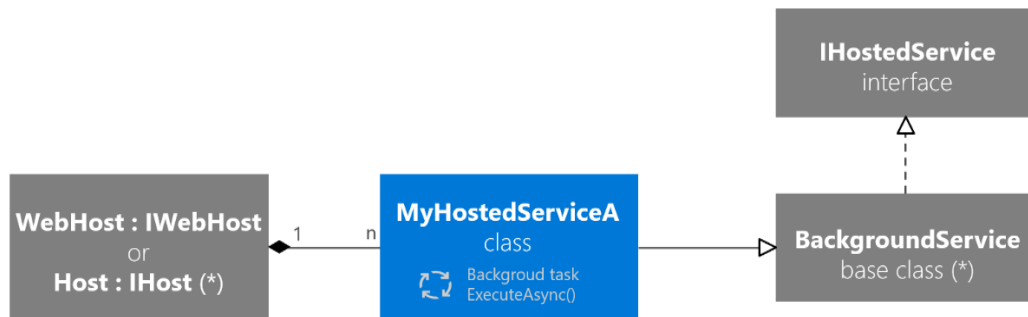
自定义 IHostedService 和相关类和接口的类图
