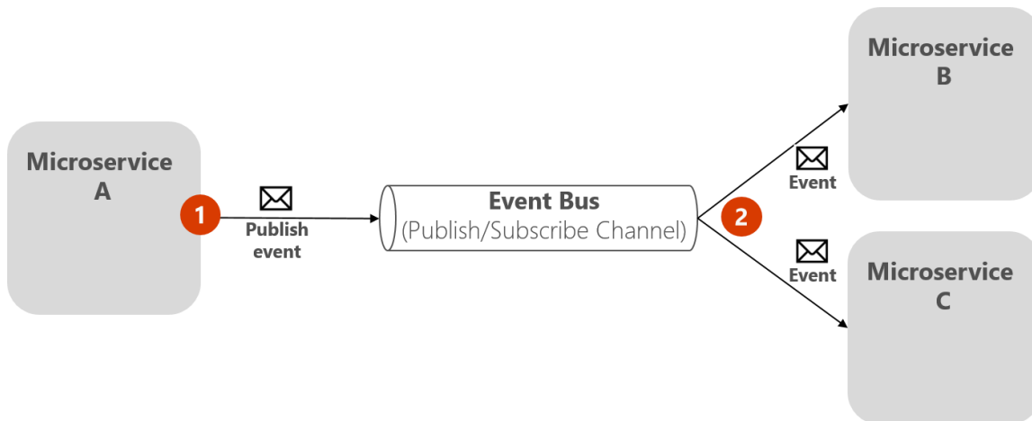
图 8-19. 使用事件总线发布/订阅的基础形式
