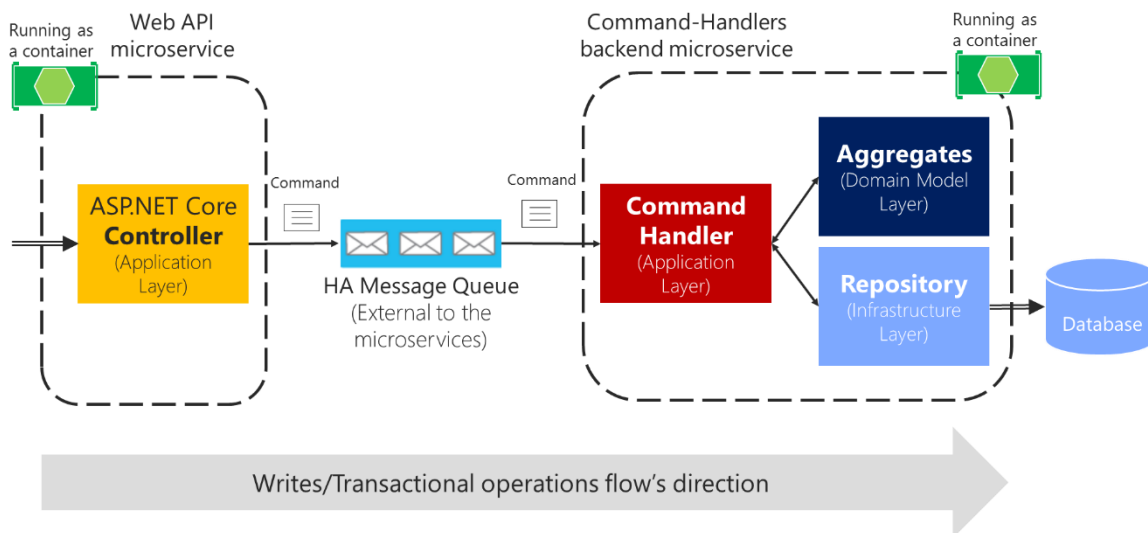
图 9-26. 使用 CQRS 命令的消息队列 (进程外通信和进程间通信)
