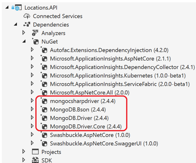
图 9-22. 在 .NET Core 项目中的 MongoDB API NuGet 包引用
