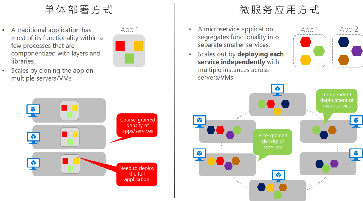
图 4-6. 单体式部署和微服务方式的对比
