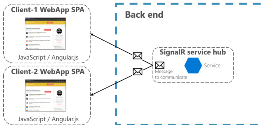
图 4-17. 一对一的实时异步消息通信
