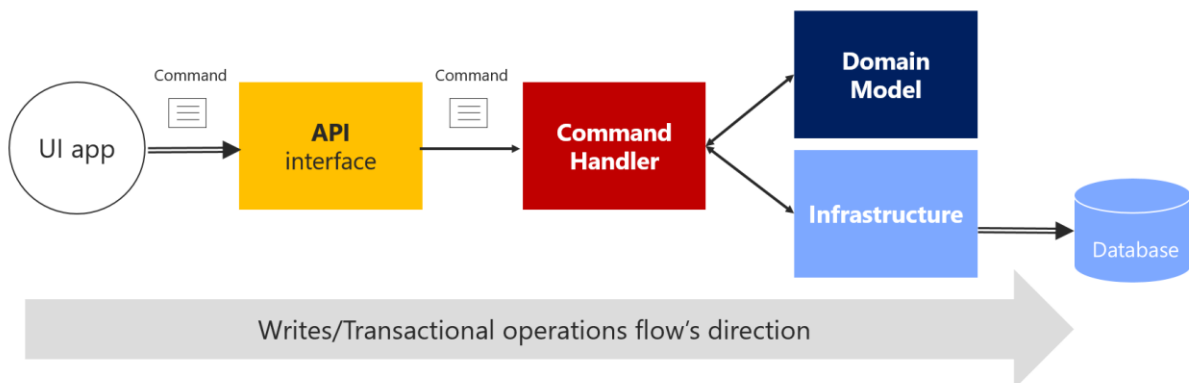
图 9-24. CQRS 模式中命令或“事务层面”的高级视图
