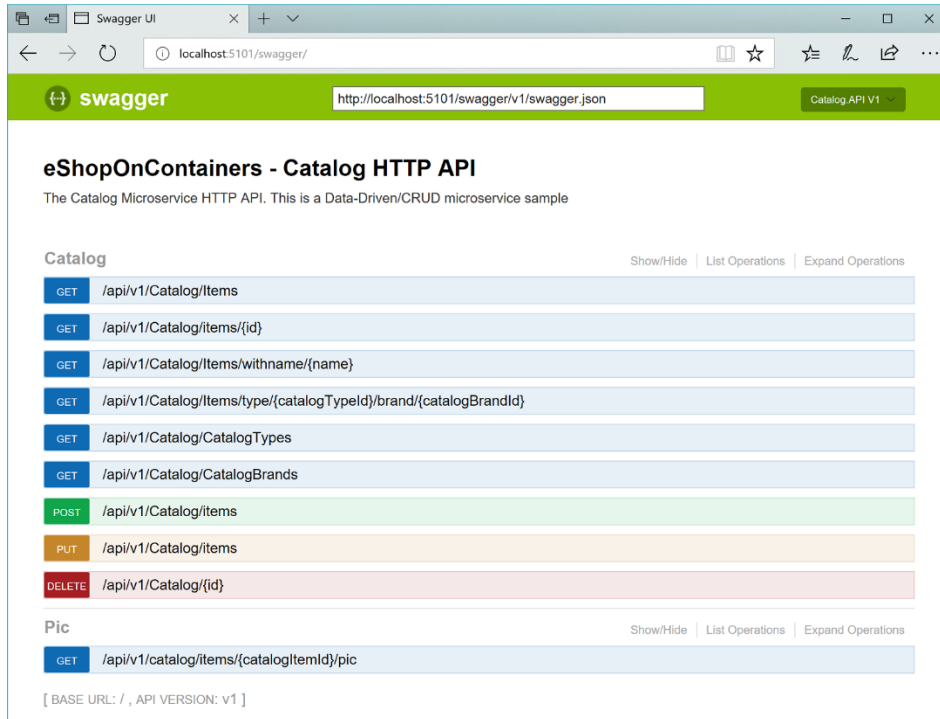
图 8-8. Swashbuckle API Explorer, 基于 Swagger 元数据的 eShopOnContainers 目录微服务
