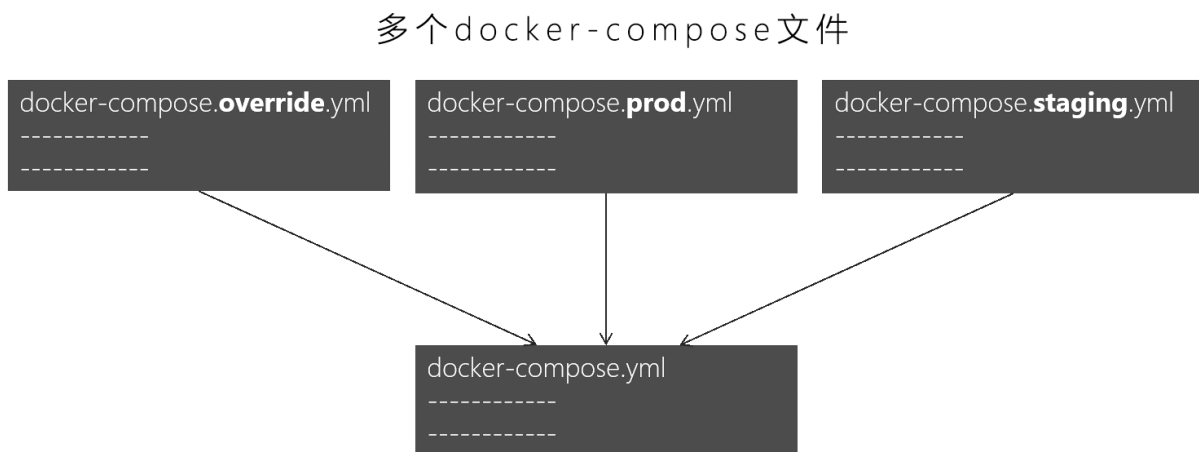
图 8-12. 多个 docker-compose 文件重写基本 docker-compose.yml 文件中的值
