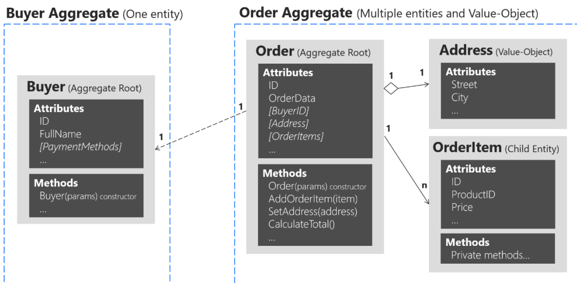
图9-9. 跟单一或多个实体聚合的例子
