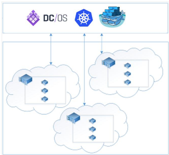
图4-25. ACS 里的编排引擎
