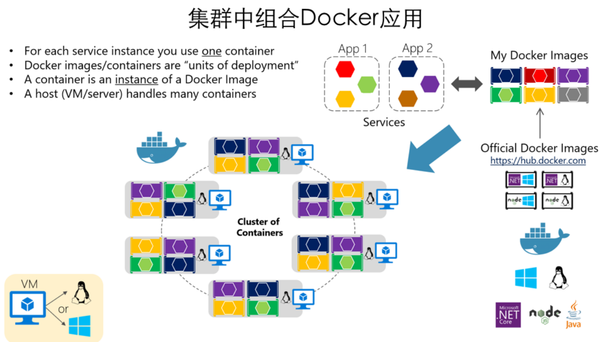
图 4-23. 一个容器集群
