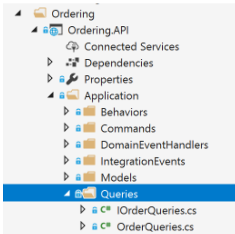
图9-4. eShopOnContainers 的订单微服务中的查询
