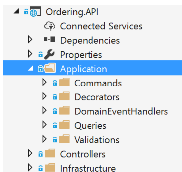
图9-23. Ordering.API ASP.NET Core Web API 项目的应用层
