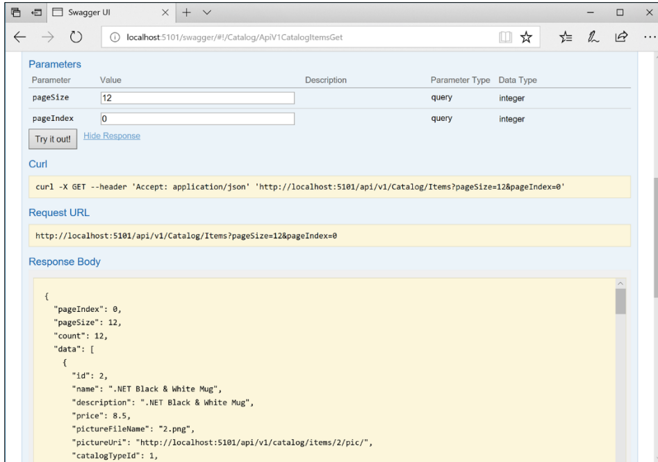
图 8-9. Swashbuckle UI 测试 Catalog/Items API 方法
