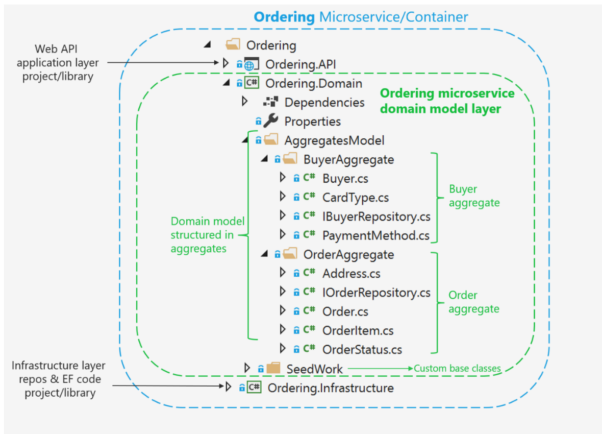
图 9-10. eShopOnContainers 中订单微服务的领域模型结构
