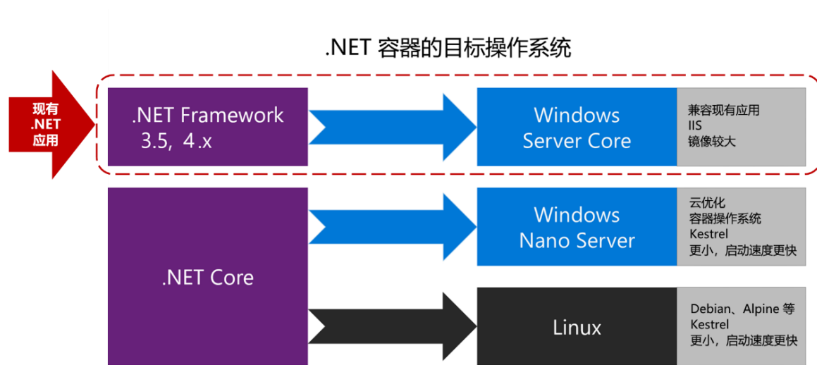
图 3-1. 根据 .NET 框架的版本来选择操作系统
