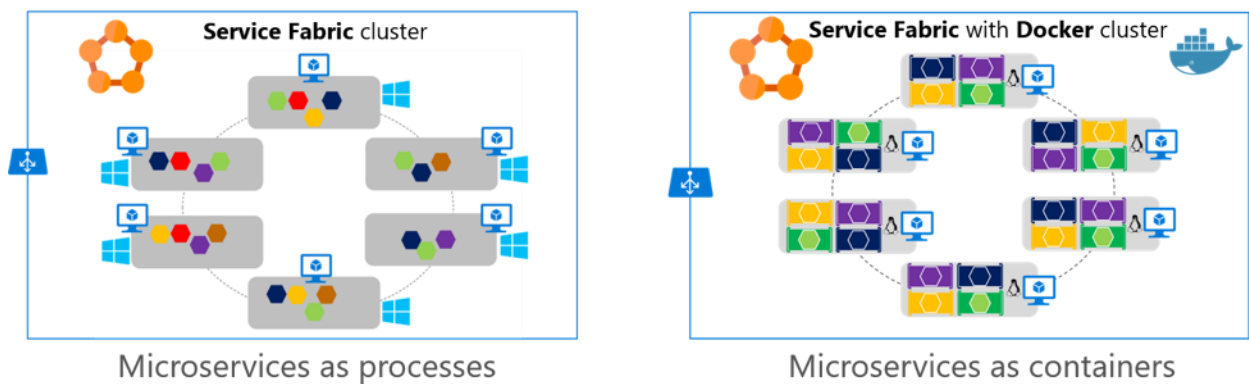
图 4-26. 在 Azure Service Fabric 以进程或容器部署微服务
