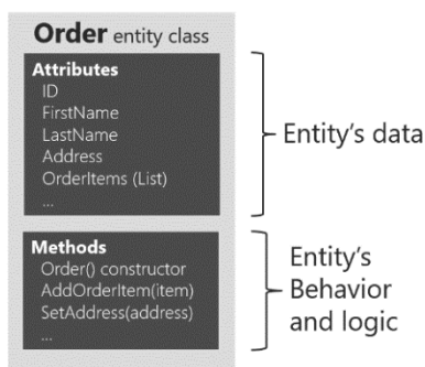
图9-8. 实现数据和行为的领域实体设计示例
