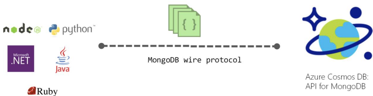
图9-20. 使用 MongoDB API 和协议访问 Azure Cosmos DB
