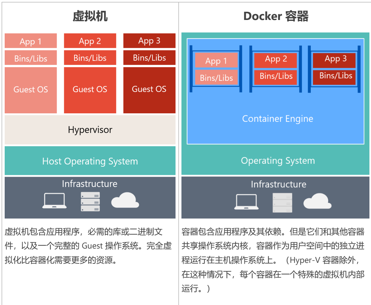
图 2-3. 传统虚拟机和 Docker 容器之间的对比
