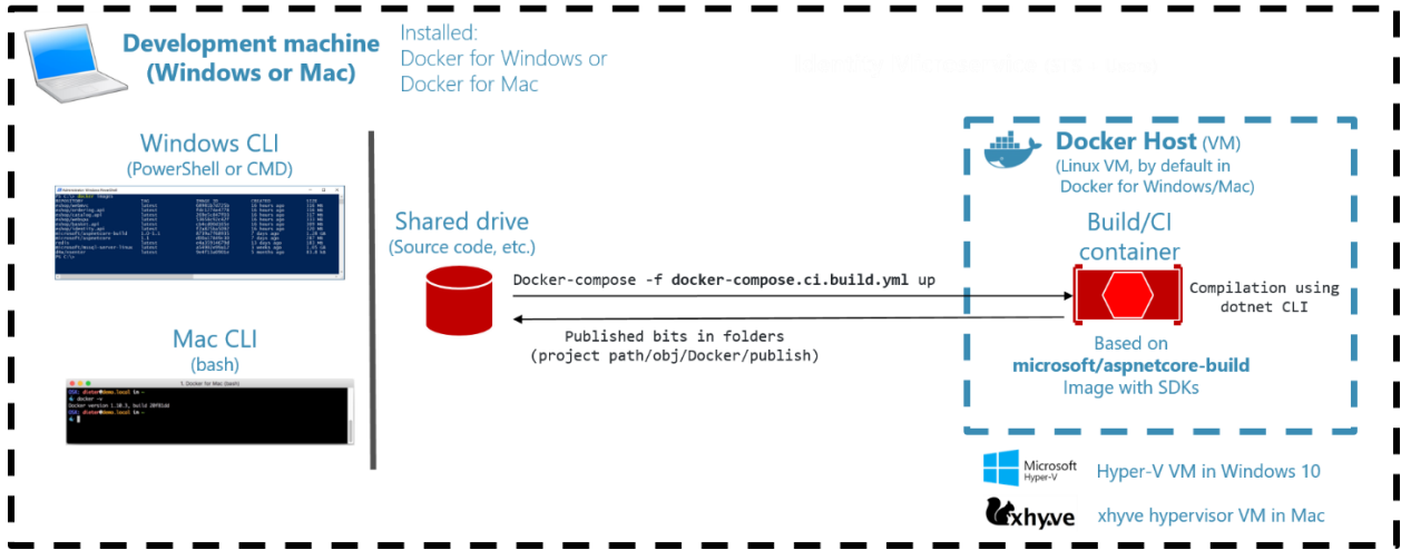
图 8-13. Docker 构建容器编译您的.NET 二进制组件
