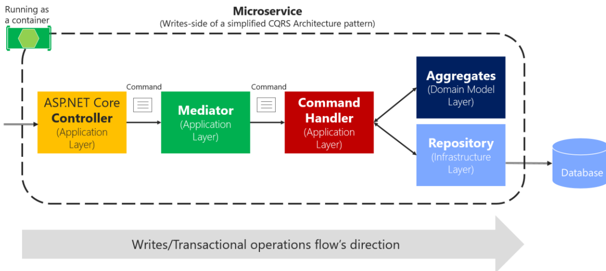
图9-25. 在单个 CQRS 微服务进程中使用中介者模式
