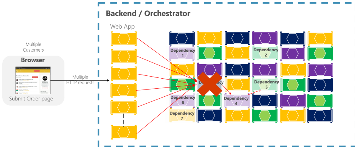
图 10-3. 具有长链的同步 HTTP 调用的微服务放大局部故障
