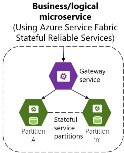
图 4-27. 使用多个有状态服务实例和一个自定义网关前端的业务微服务
