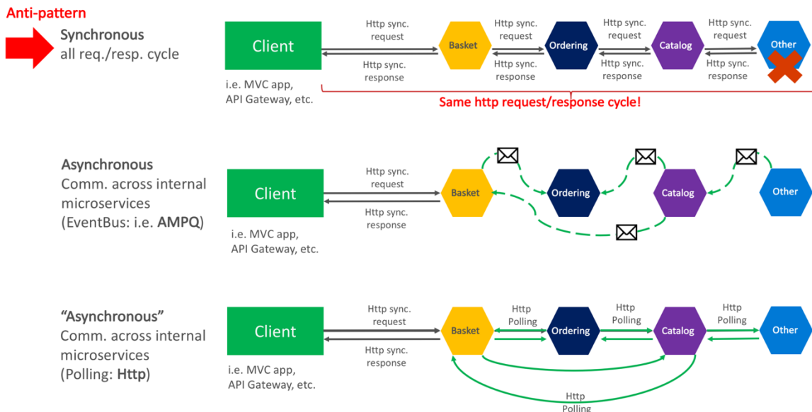
图 4-15. 微服务通信的反模式和模式
