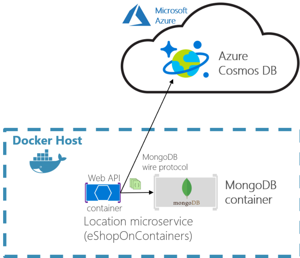
图9-21. eShopOnContainers 使用 MongoDB 容器用于开发环境或者产品的 Azure Cosmos DB 环境
