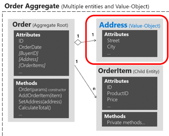
图9-13. Order 聚合中的 Address 值对象
