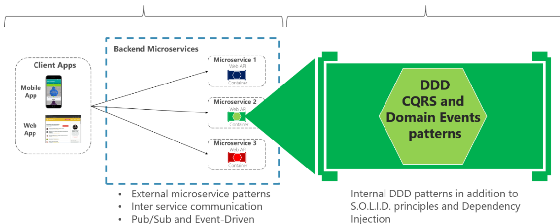
图 9-1. 应用外部微服务架构与微服务内部架构模式
