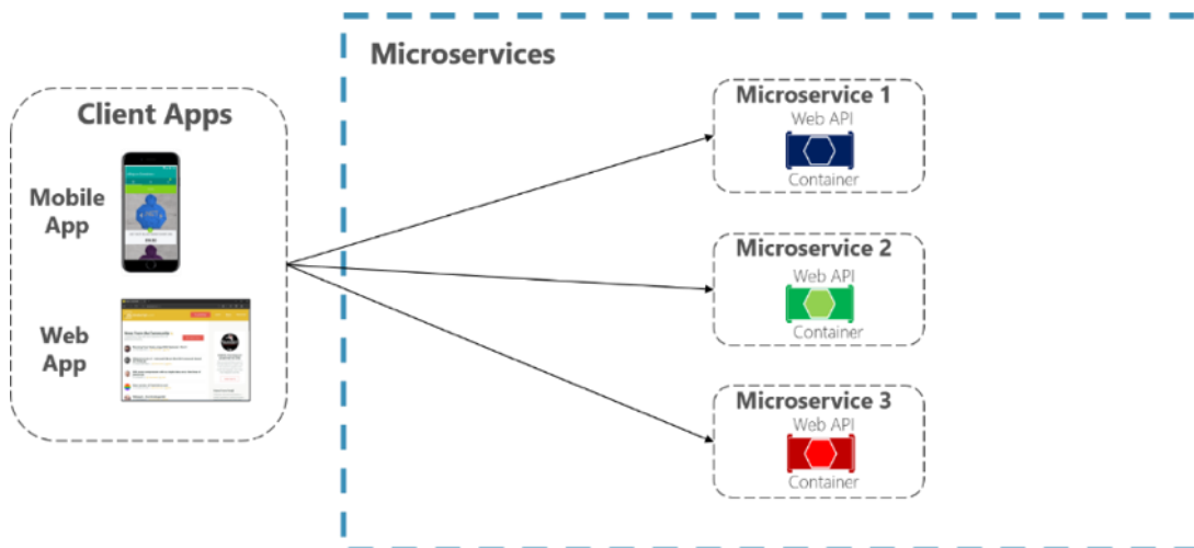
图 4-12. 使用客户端微服务直连的架构
