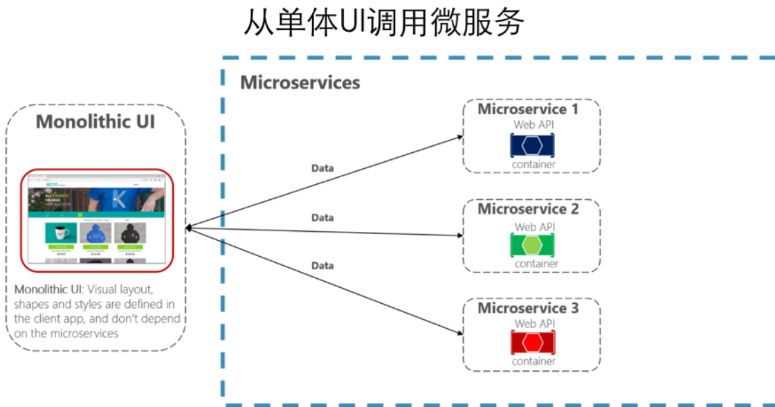
图 4-20. 一个调用多个后台微服务的单体 UI 应用
