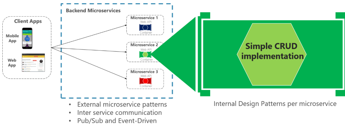
图 8-4. 简单的 CRUD 微服务的内部设计
