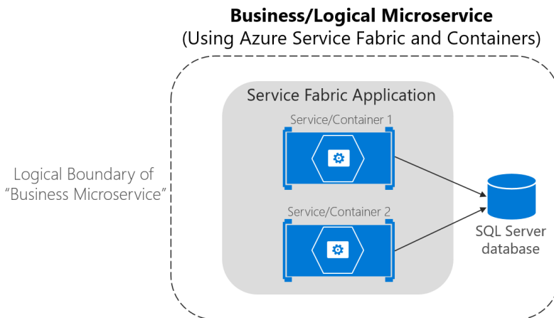
图 4-28. 在 Service Fabric 中使用多个服务（容器）的业务微服务
