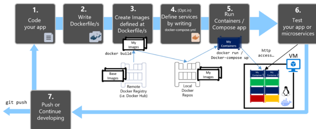
图5-1. 开发 Docker 容器化应用程序的步骤
