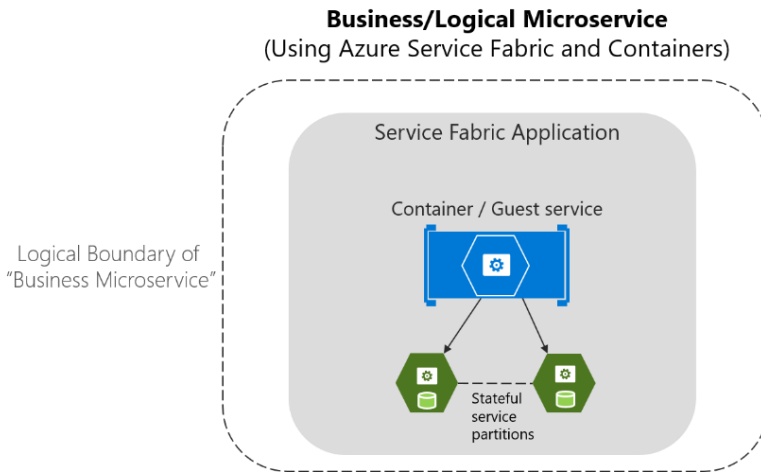
图 4-29. 使用容器和有状态服务映射到一个 Service Fabric 应用的业务微服务
