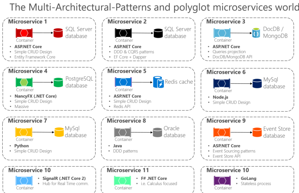
图 8-3. 多种架构模式和多语言的微服务世界
