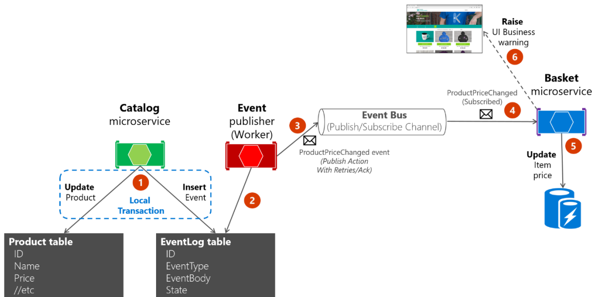
图 8-23. 使用一个 Worker 微服务将事件发布到事件总线时的原子性
