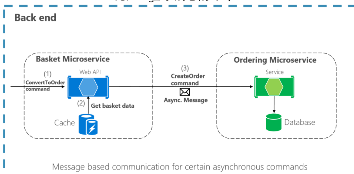
图4-18. 一个接收异步消息的微服务
