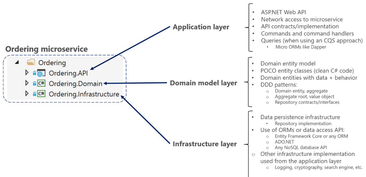
图 9-5. eShopOnContainers 里订单微服务中的 DDD 分层
