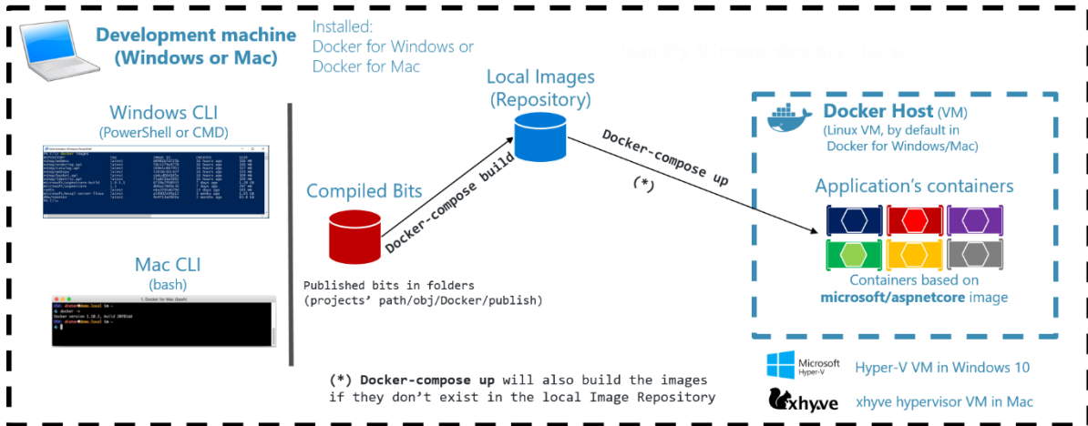
图 8-16. 构建 Docker 镜像并运行容器
